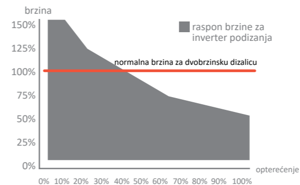
Dijagram opterećenja i brzine u tehnologiji invertera dizanja
